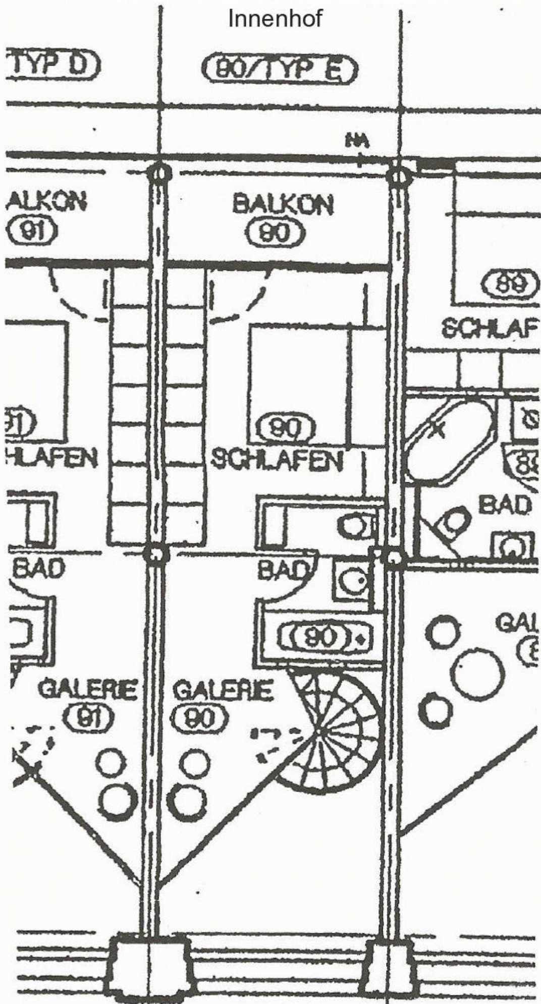
Grundriss 2. Zwischengeschoss (obere Ebene)
